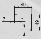
Уголок внешний (Тип 2) К32
