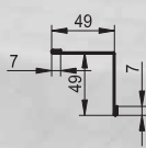
Уголок внутренний (Тип 2) KB2
