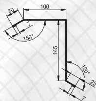
Ветровая защита (Тип 2) ВЗ2
