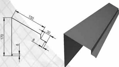
Полукопек плоский НКП
