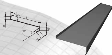
Конек плоский (Тип 1) КП1
