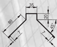
Конек плоский (Тип 2) КП2
