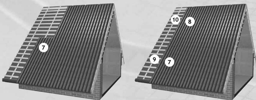
Рис. 22. Последовательность устройства рядовых листов
