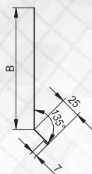
Конек универсальный КУ
