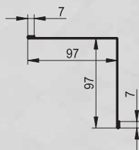
Уголок внутренний (Тип 2) KB2
