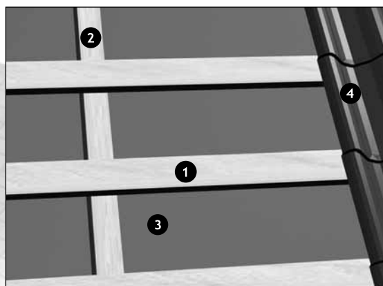
Рис. 6. Конструкция обрешетки
